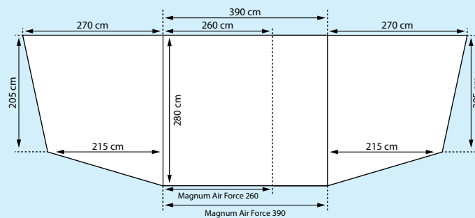
Afmetingen Magnum Air Force 390
